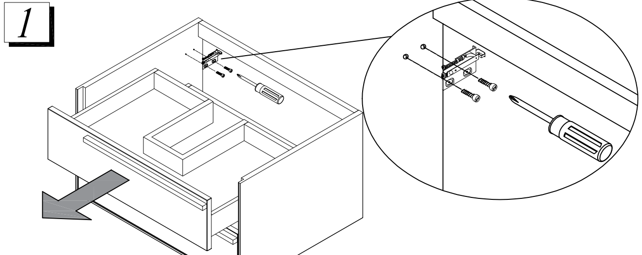
Demontaža / Dissmounting
